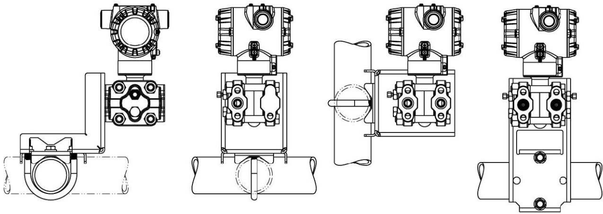
安装构造
